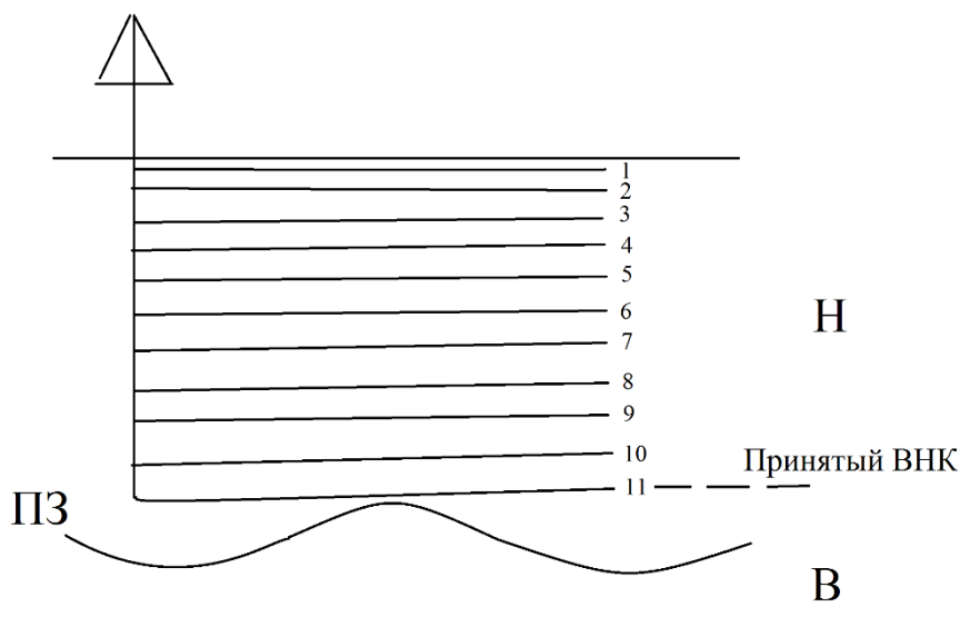
Рис.1. Схематичное расположение горизонтального участка скважины в интервале пласта; ствол на удалении от кровли 1 – 7,5%; 2 – 10%; 3 – 12,5%; 4 – 25%; 5 – 40%; 6 – 50%; 7 – 60%; 8 – 70%; 9 – 80%; 10 – 90%; 11 – 100% (на уровне принятого ВНК); Н – нефтяная зона; ПЗ – переходная зона; В – водная зона
