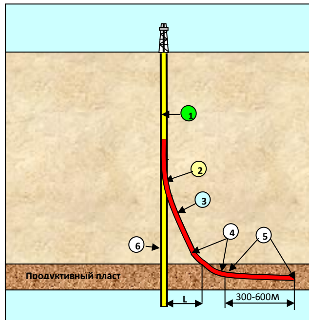
Рис. 1. Схема профиля горизонтальной скважины
